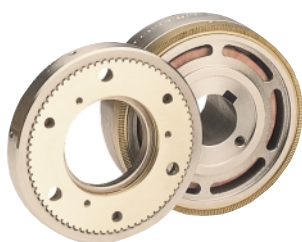
INNESTI ELETTROMAGNETICI A DENTI COPPIE FINO A 2200 (Nm) (disponibile solo scheda)
